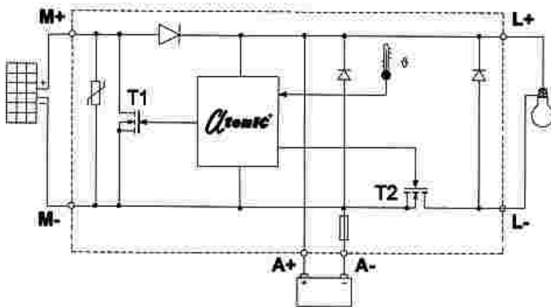
Рис. 1. Принципиальная схема контроллера
