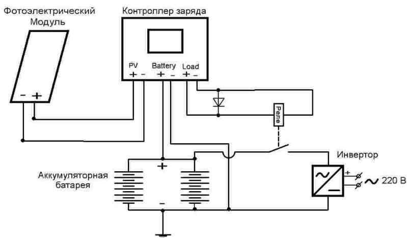
Рис. 3 Схема подключения инвертора в системе
