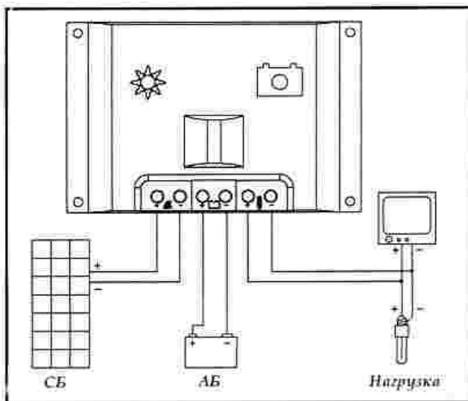
Рис. 2. Схема соединений
